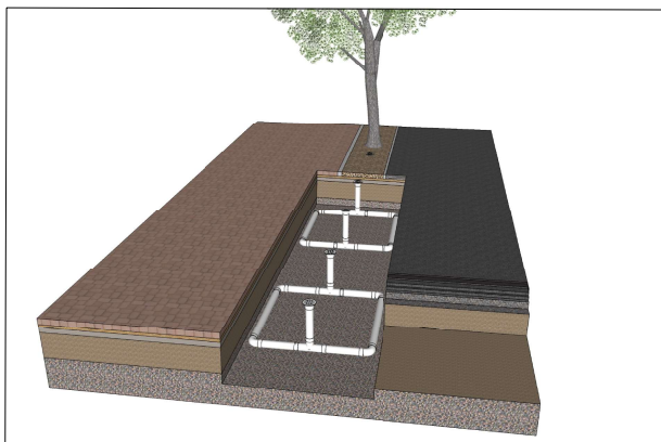
Principe beluchtingsdrain
