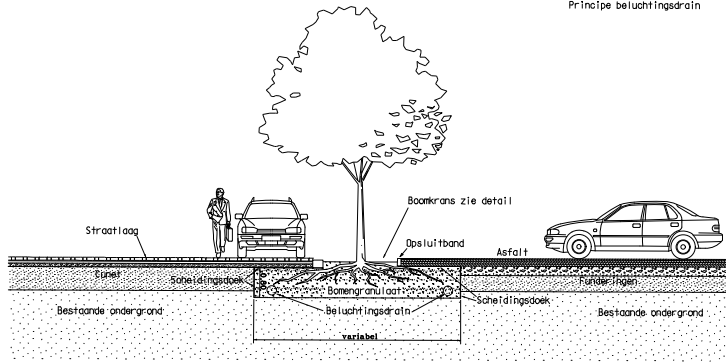
Principe beluchtingsdrain
